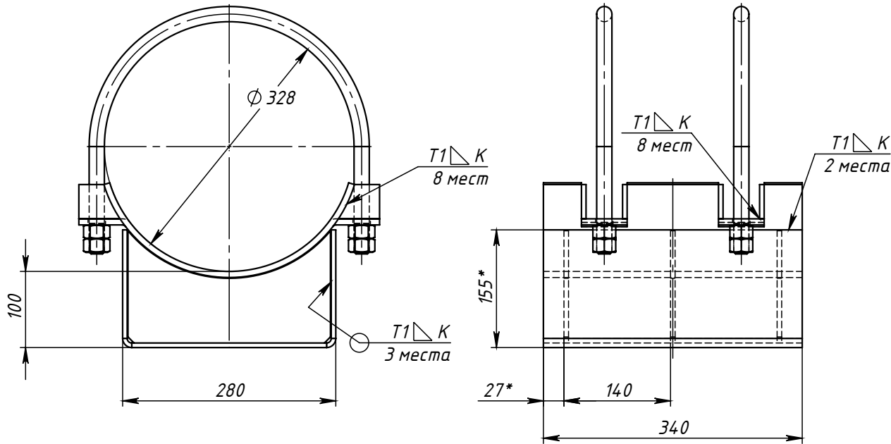
Поз.3 (Ложемент)
