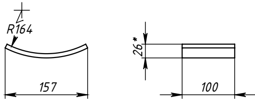
Поз.6 (Упор)
