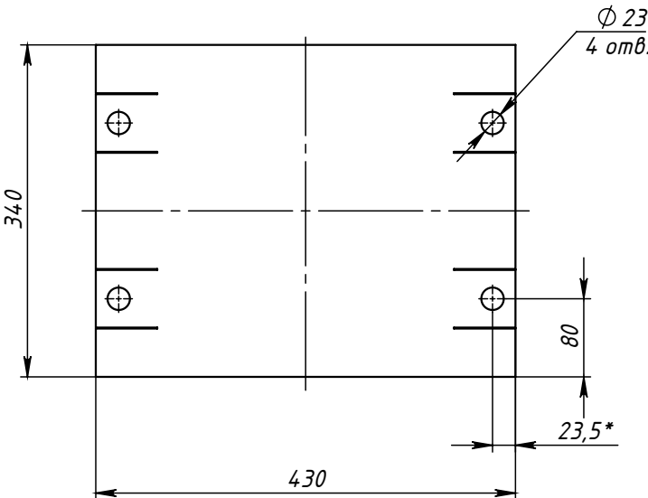
Поз.3 (Ложемент) развертка
