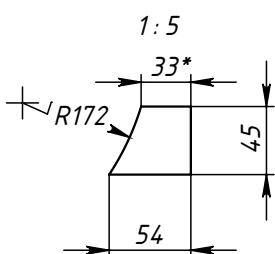
Поз.4 (Косынка)
