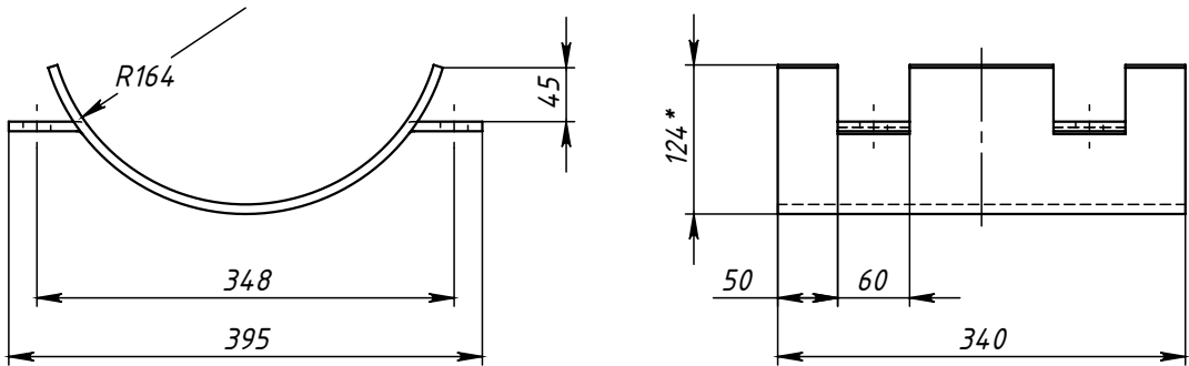
Поз.3 (Ложемент)
