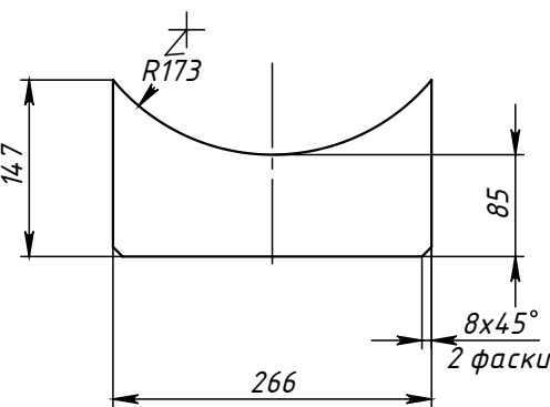
Поз.2 (Ребро)
