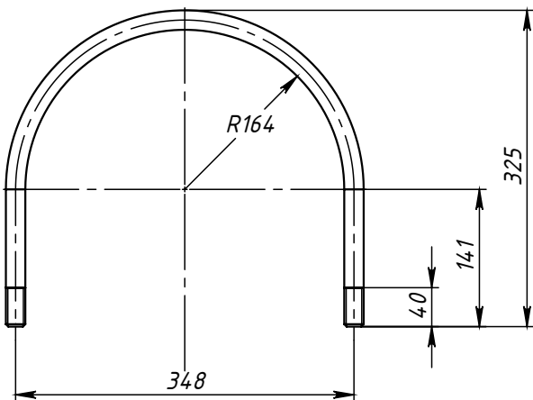
Поз.5 (Хомут)
